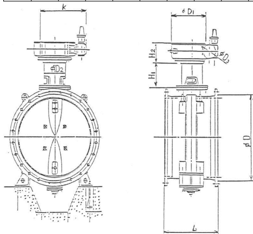
◎制水（蝶形）弁（Ⅱ） B 4 1, B 4 4, B 5 2
