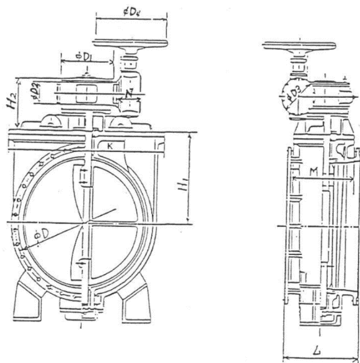
◎制水（蝶形）弁（Ⅰ） B 4 2
